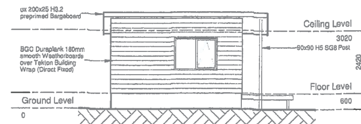
2 Elevation 1 1 : 100
