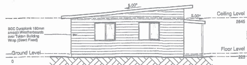
3 Elevation 4 1:100
