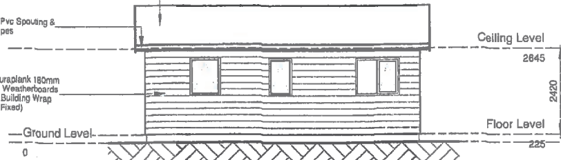
2 Elevation 1 1 : 100
