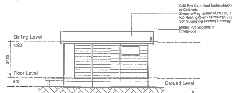
5 Elevation 3 1 : 100
