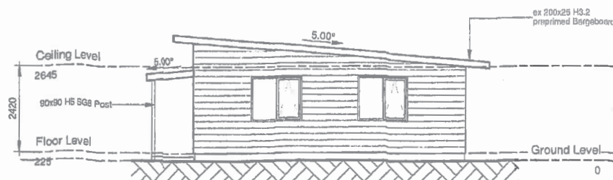
2 Elevation 2 1:100
